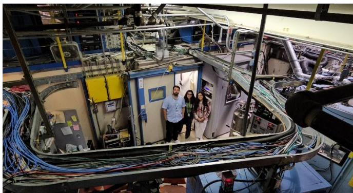
Figura 2. Estación experimental para absorción de rayos X (línea 7-3) en el sincrotrón SSRL del laboratorio nacional SLAC de la universidad de Stanford.
